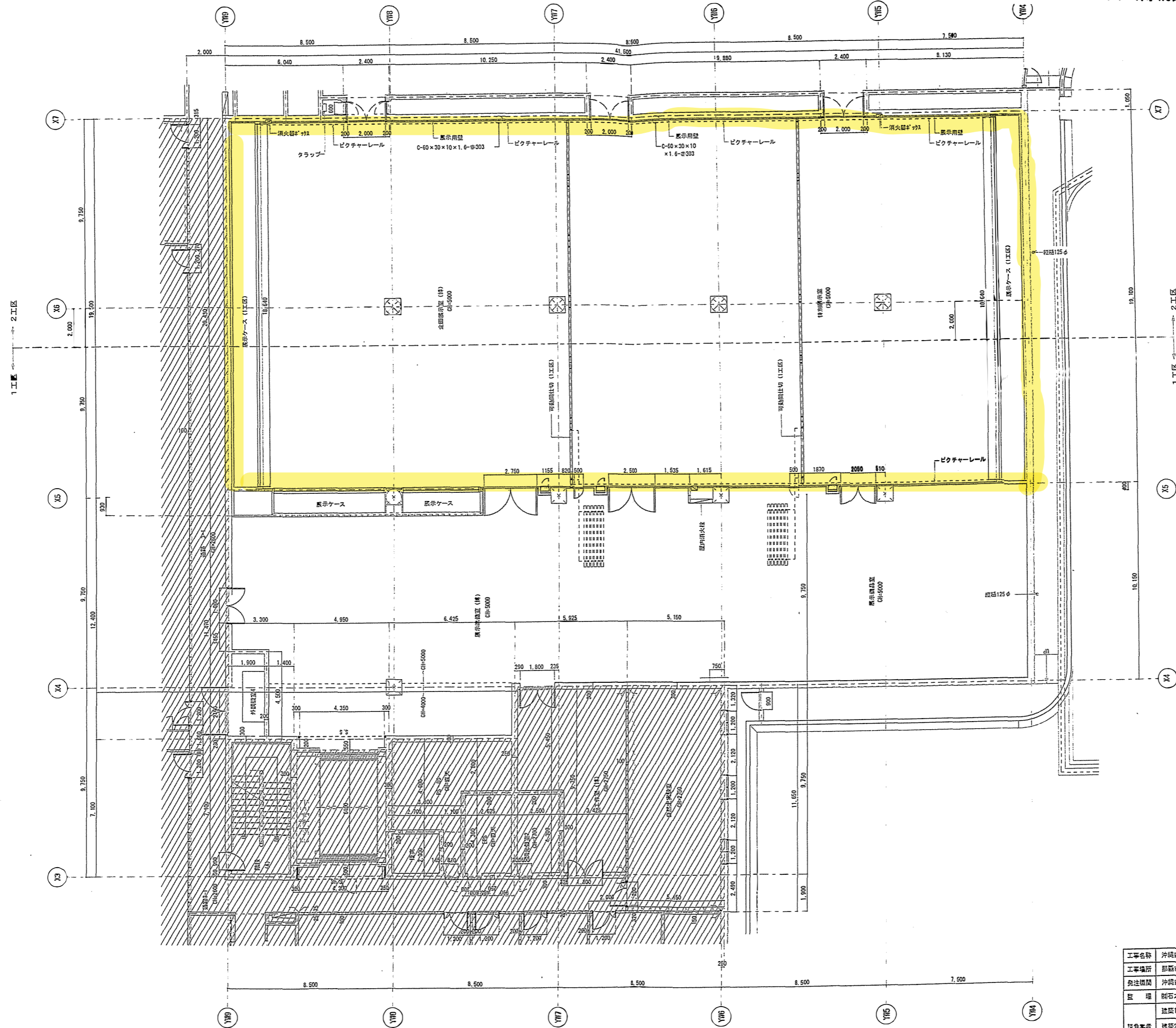
展示室配置がわかる図面 (博物館特別展示室企画展示室平面図)
