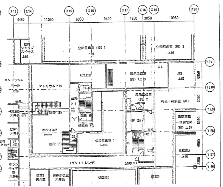
2階平面図 (1FL+3.600)
